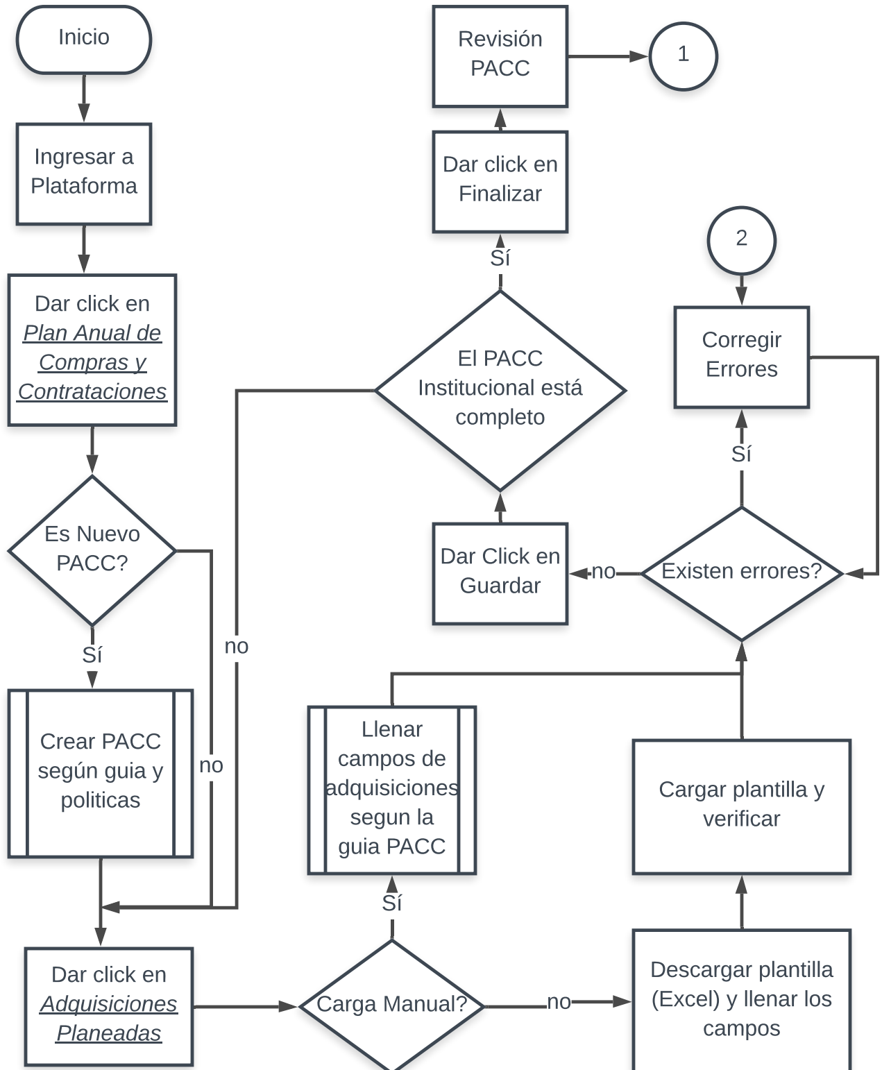
Honducompras 2.0 Diagrama de Flujo: Flujo Elaboración PACC
