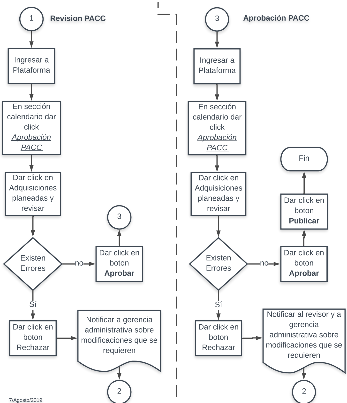
Honducompras 2.0 Diagrama de Flujo: Flujo Elaboración PACC
