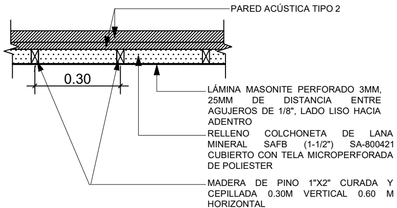
4 DETALLE PANEL ACÚSTICO
