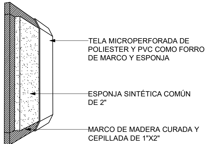
5 DETALLE PÁNELES DE ESPONJA SINTÉTICA
