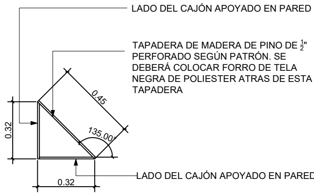
1 VISTA EN PLANTA TRAMPA DE BAJOS
