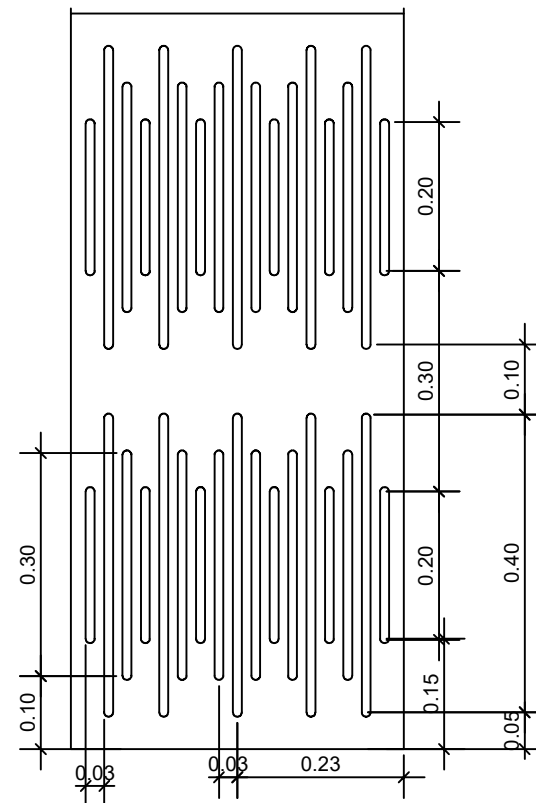
3 PATRÓN DE PERFORADO TRAMPA DE BAJOS
