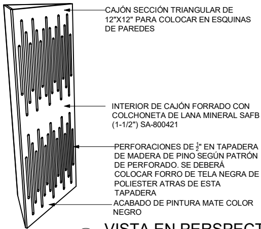
2 VISTA EN PERSPECTIVA TRAMPA DE BAJOS
