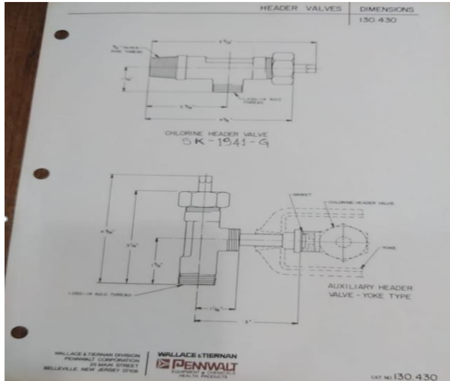
Detalle válvulas en línea
