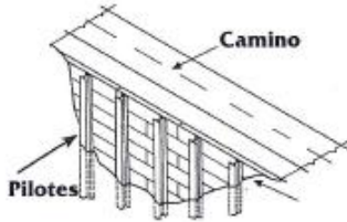
Cabezales
