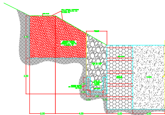
DETALLE 'A' ESCALA 1:30
