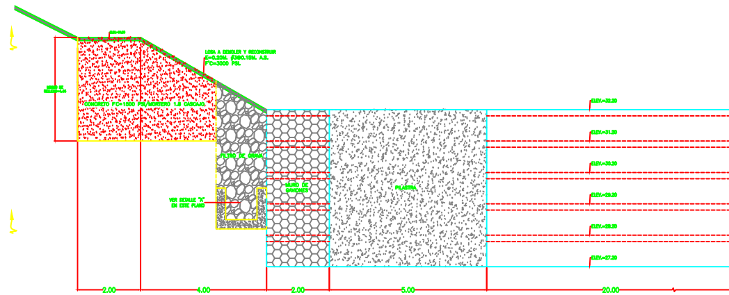
SECCION 1-1 ESCALA 1:50
