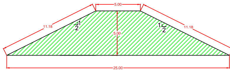
SECCION TIPICA MARGEN DERECHA DEL RIO ULUA
