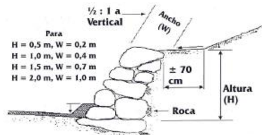
Relleno de agregados Roca
