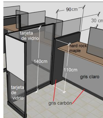
Ilustración 1 Mampara toma de fotografías
