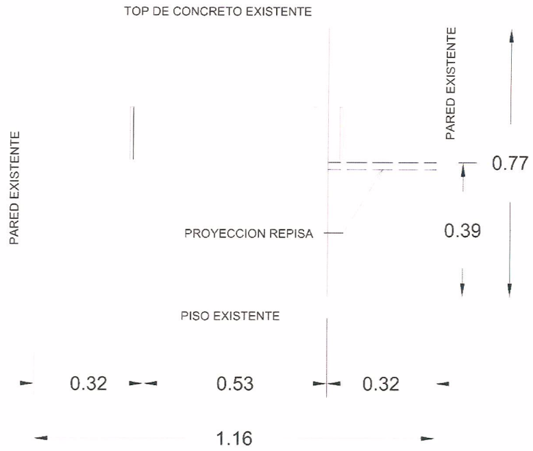
DETALLE DE MUEBLE DE COCINA
