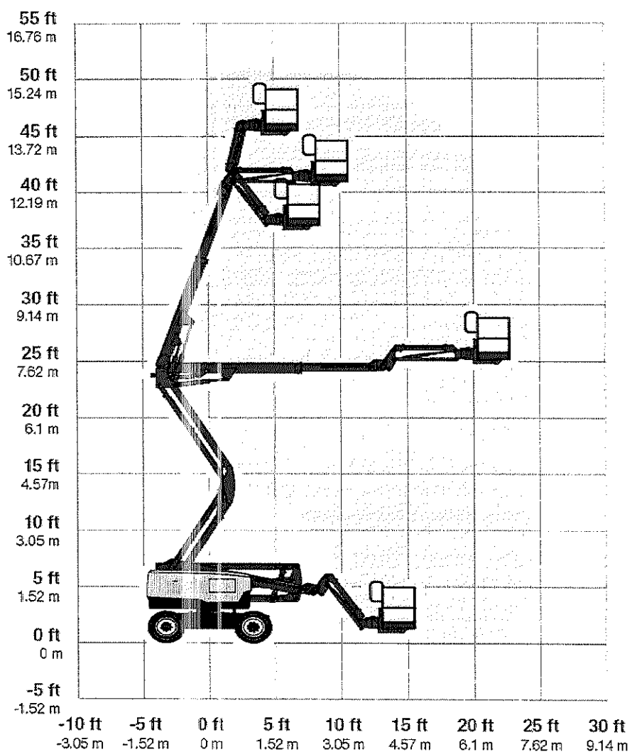
Figura 1. Rangos de movimientos requeridos para la Plataforma Elevadora Autopropulsada.
