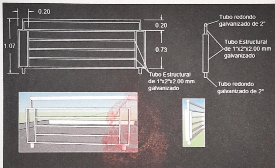
Detalle de baranda en rampa y área de terraza
