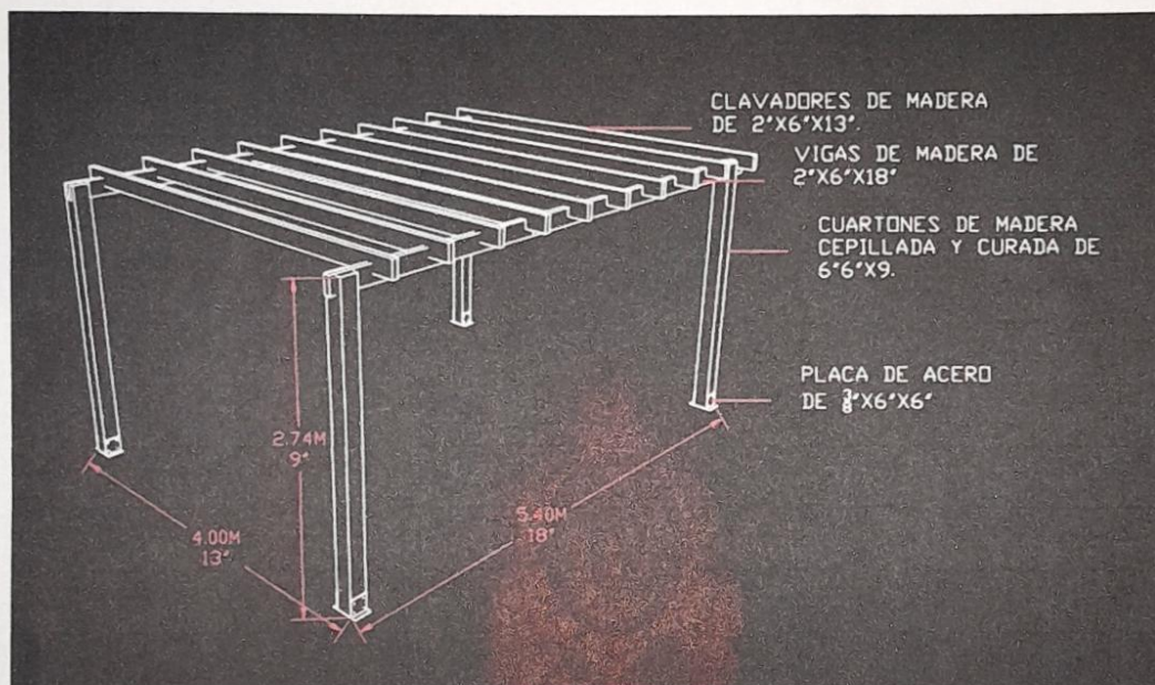
DETALLE DE PERGOLA (toda la madera es cepillada curada).
