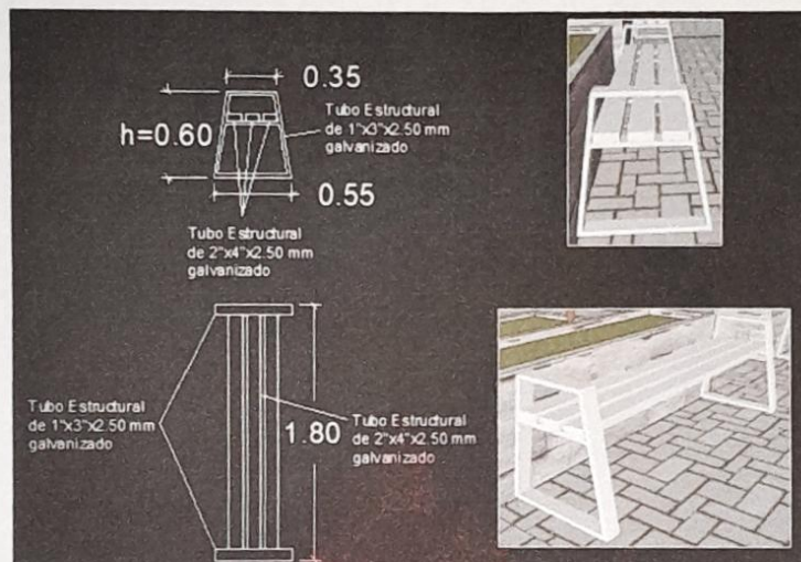
IMAGEN 2-2: Detalle de banca
