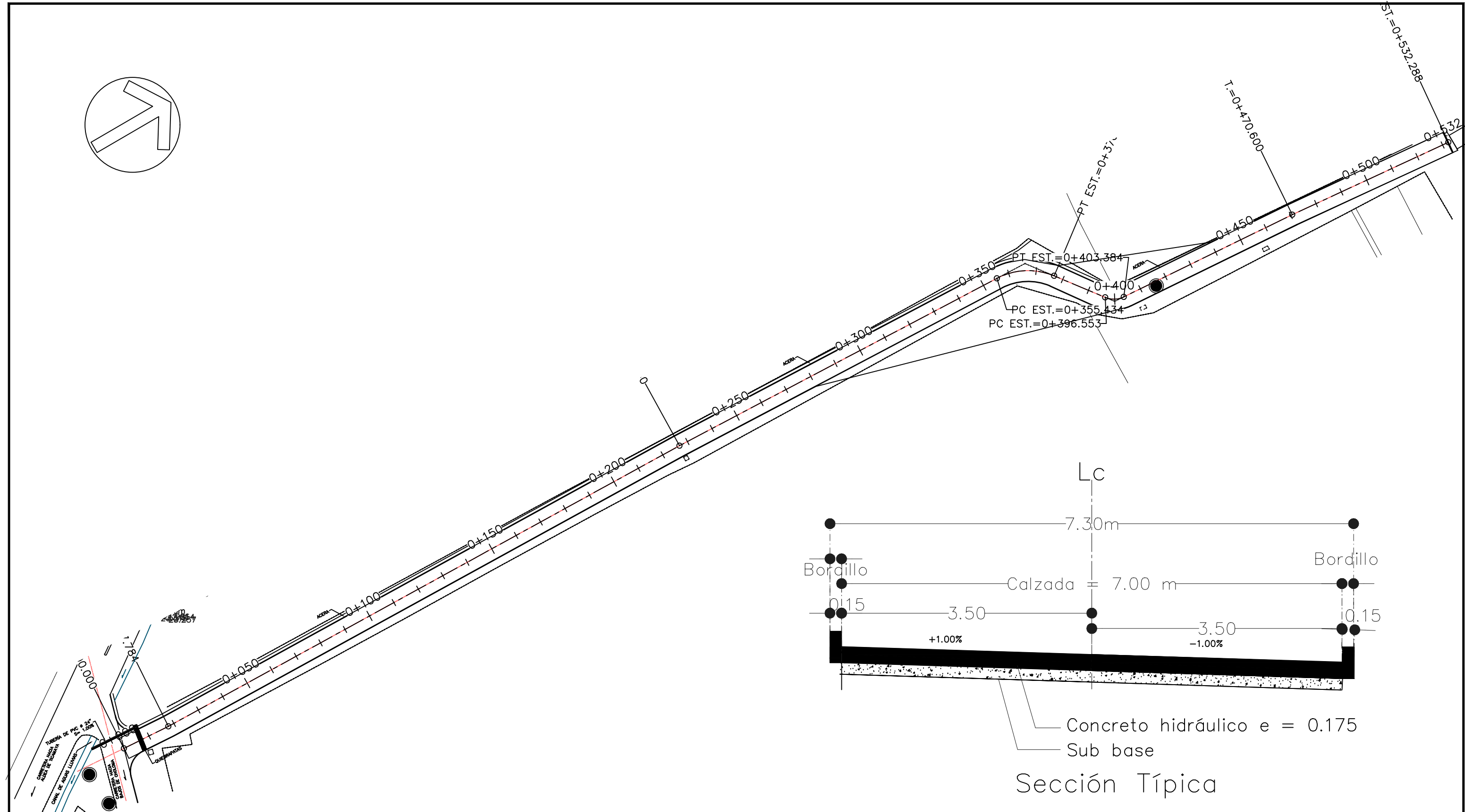
PERFIL GENERAL DE LA EST 0+000 A LA EST 0+532
