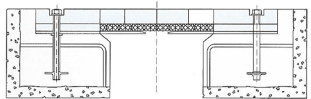
Fig. 3: Tipo 3 con perfil de elastómero.
