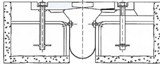
Fig. 2: Tipo 2 con babero en forma de lira.
