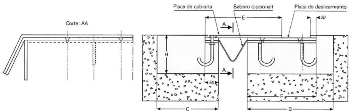
Fig. 1: Junta de acera.
