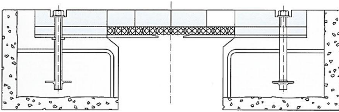
Fig. 3: Tipo 3 con perfil de elastómero.
