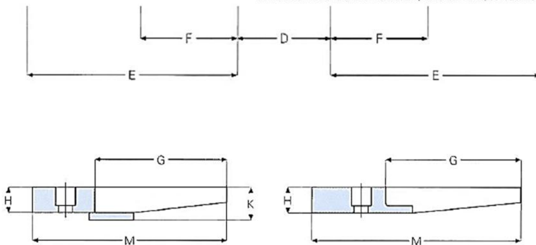
Arriba: WP estándar. Al lado: WP de aleación de aluminio.
