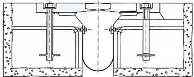
Fig. 2: Tipo 2 con babero en forma de lira.
