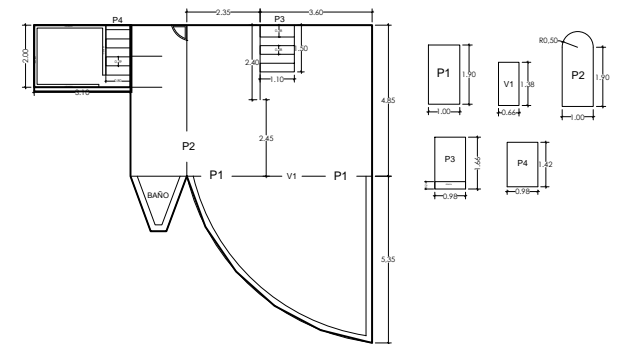
DETALLE INTERIOR BAJO MIRADOR (BAÑOS)
