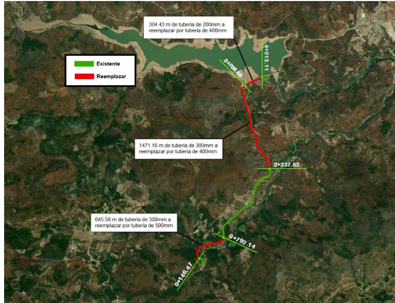
Esquema de Reemplazo de tubería
