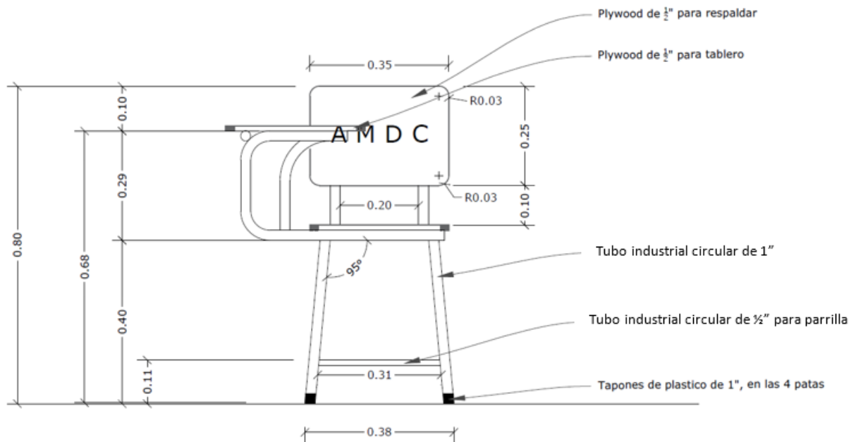
VISTA FRONTAL DE PUPITRE
