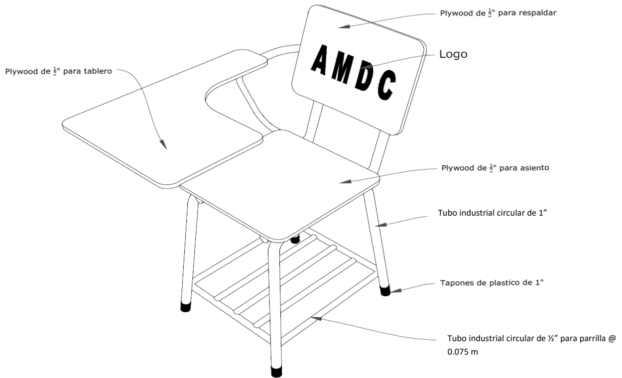
DETALLE DE PERSPECTIVA DE PUPITRE
