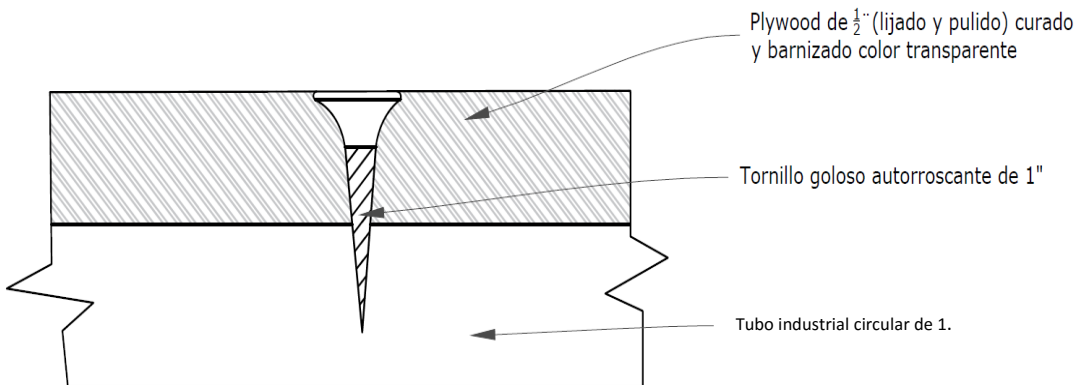
DETALLE DE ENSAMBLE DE TORNILLO
