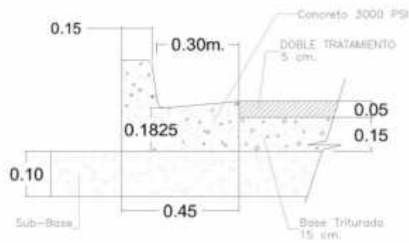
DETALLE DE BORDILLO DE CONCRETO CON CUNETTA INTEGRADA
