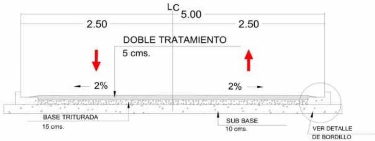
SECCION TIPICA DE DOBLE TRATAMIENTO
