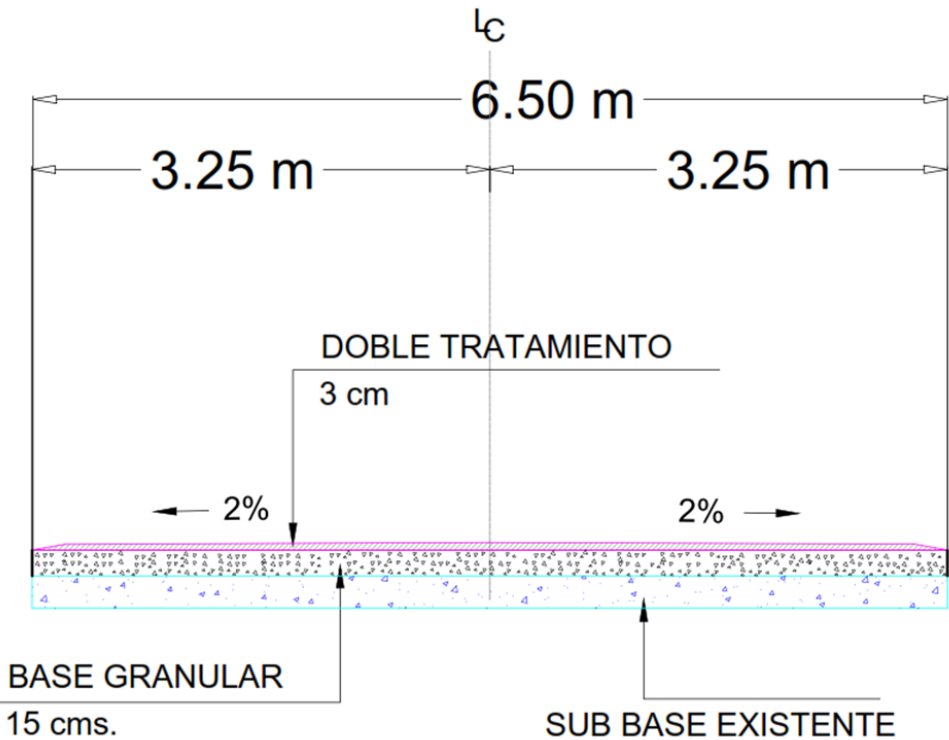
SECCION TIPICA
