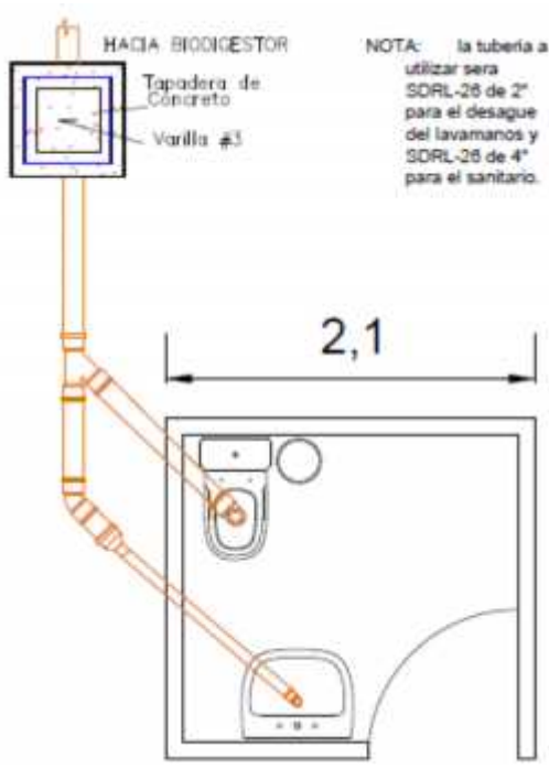
Sistema Sanitario
