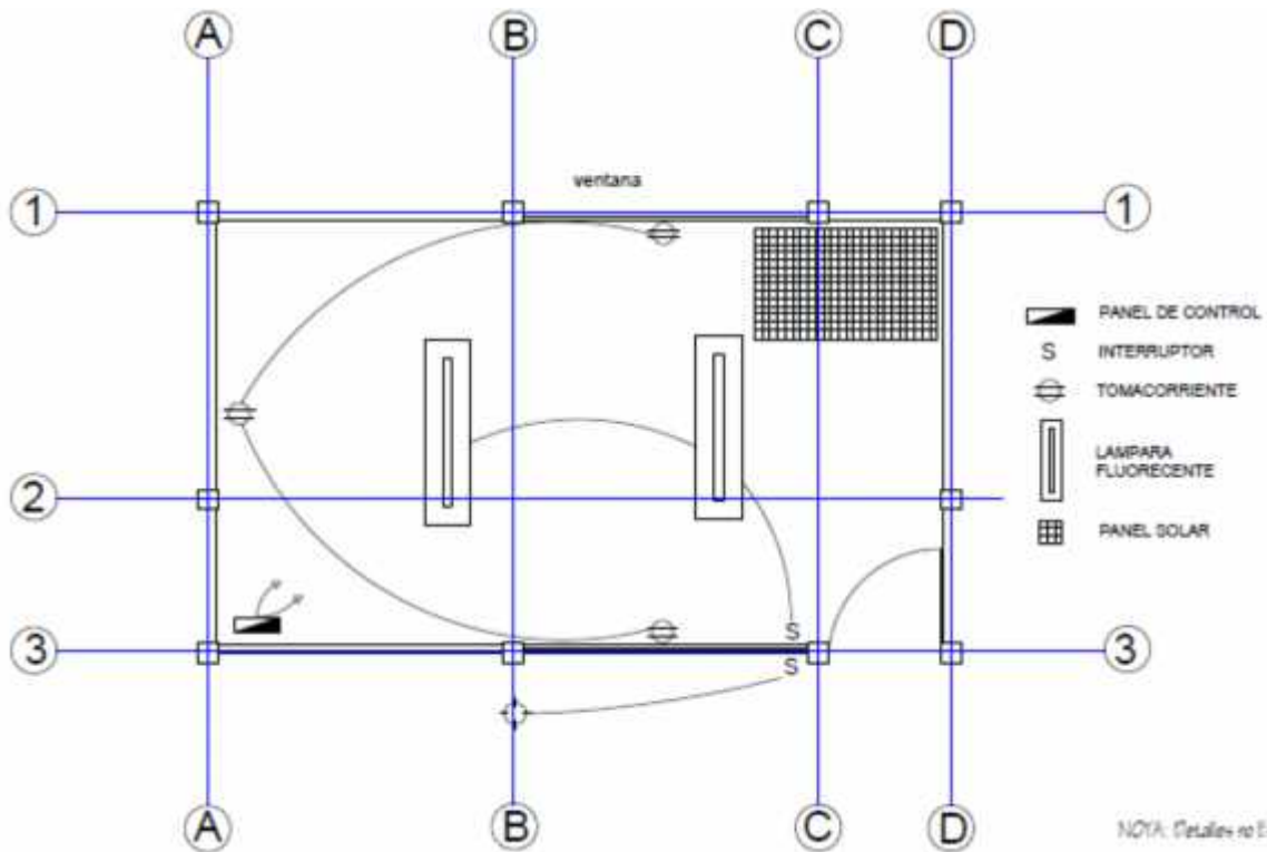
Sistema Eléctrico
