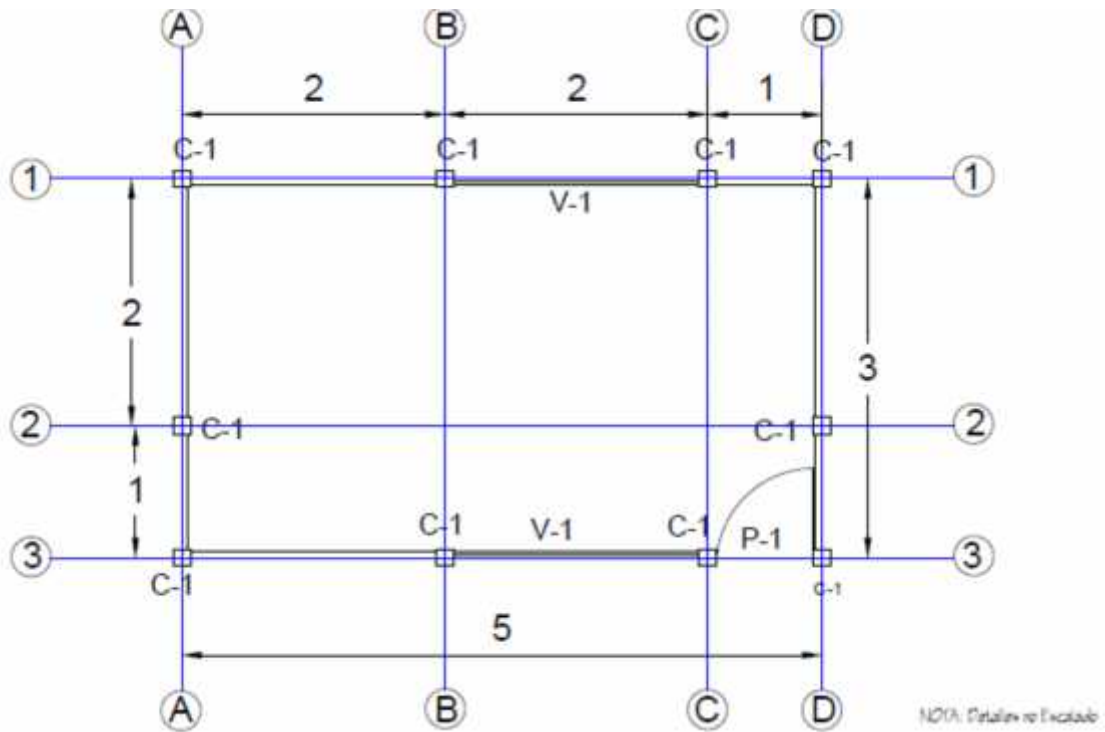
Plano Constructivo
