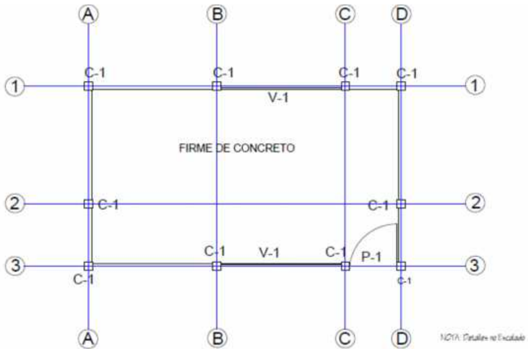
Plano Estructural
