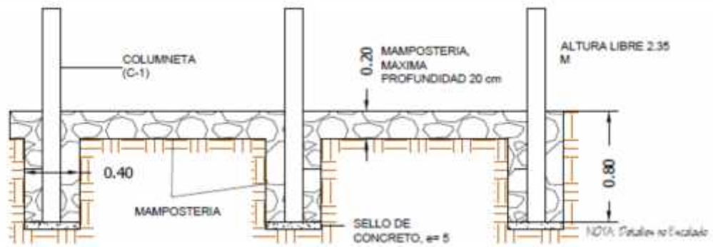
Detalle de Cimentación
