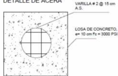
Detalle de Acera y Firme de Concreto
