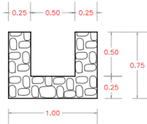
DETALLE CUNETA MAMPOSTERIA 1:30
