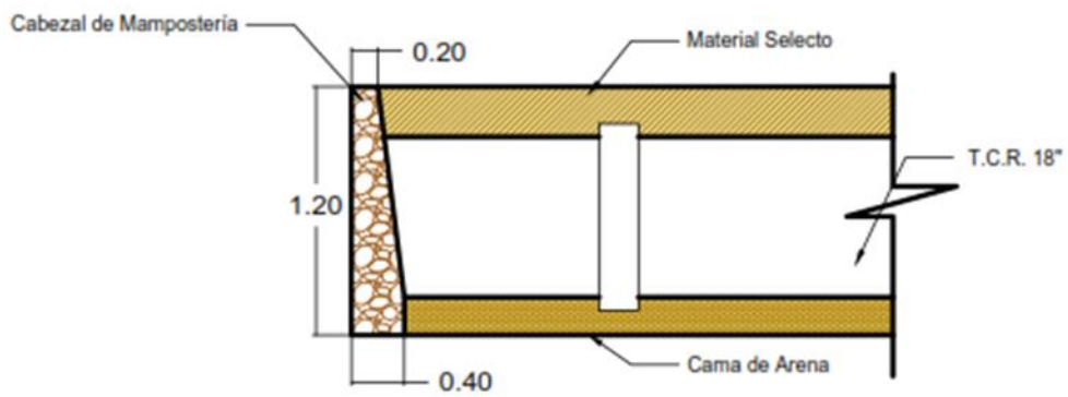
DETALLE DE CABEZAL DE MAMPOSTERÍA SIN EBOLA
