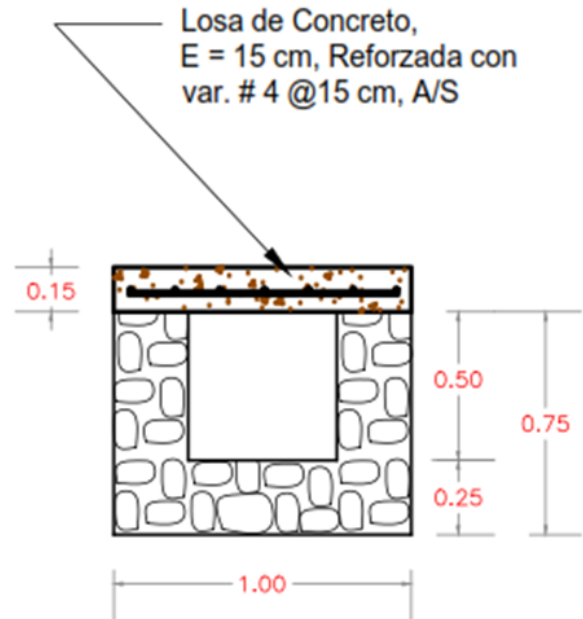
DETALLE DE LOSA DE CONCRETO SOBRE CUNETA EN CRUCE DE CALLES 1:30
