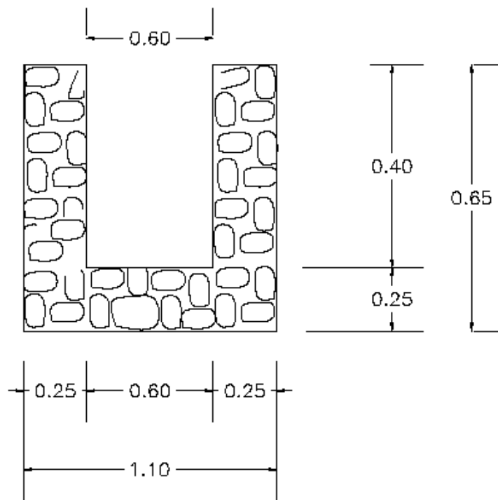
DETALLE CUNETAS DE MAMPOSTERÍA
