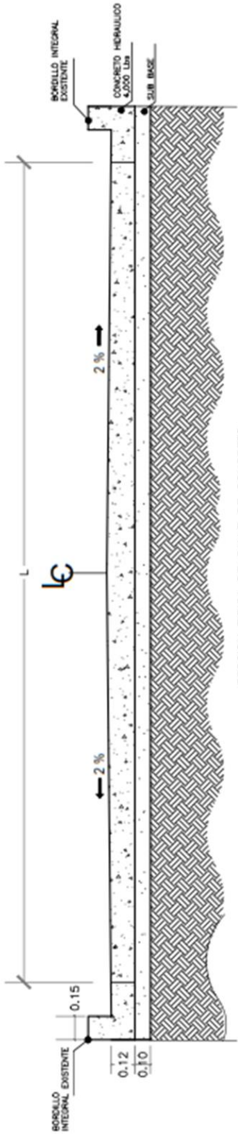
SECCION TIPICA DE CALLE DE CONCRETO HIDRAULICO CON BORDILLOS EXISTENTES. sin escoba
