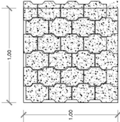
PLANTA DE ADOQUINES.
