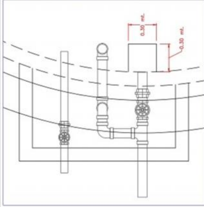
DETALLE DESAGÜE DE LIMPIEZA ESCALA 1:20
