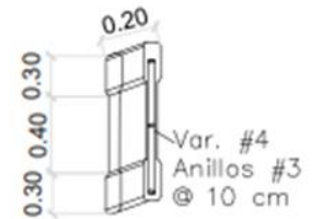
Vista isométrica
