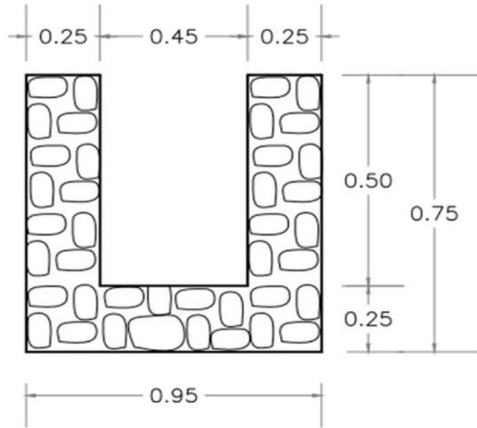
DETALLE CUNETAS
