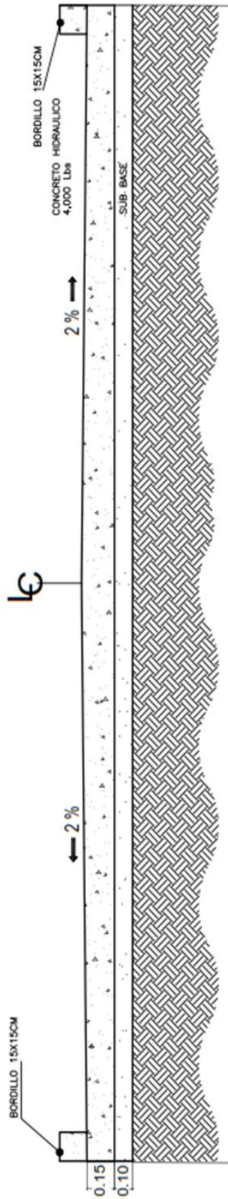
SECCION TIPICA CALLE DE CONCRETO HIDRAULICO
