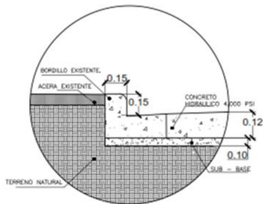
DETALLE BORDILLO DE 15 CM X 15 CM
