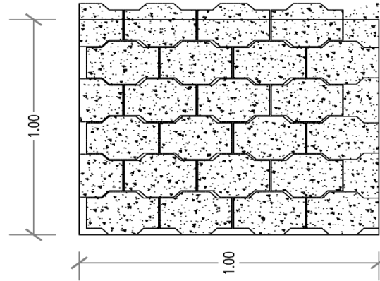
PLANTA DE ADOQUINES.
