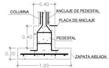
PEDESTAL DE CONCRETO DE 40 CM X 40 CM
