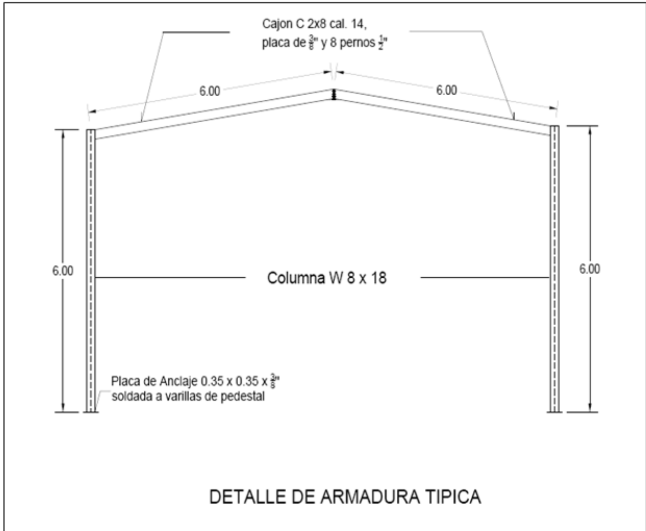
Anexo B – Armadura en Escuela Moisés Starkman
