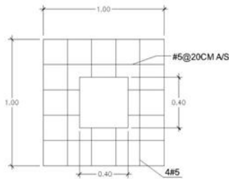
ZAPATA AISLADA 1.00X1.00X0.20M
