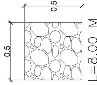
DETALLE DE CORONA PARA MURO EXISTENTE L=8.00 M
