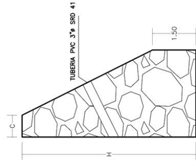
DETALLE DE MURO DE CONTENCIÓN DIMENSIONES: H=5.00 M, B=2.00 M, C=0.50 M, L=7.00 M
