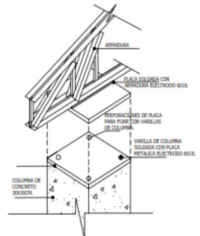
ISOMETRICO DE APOYO FIJO
