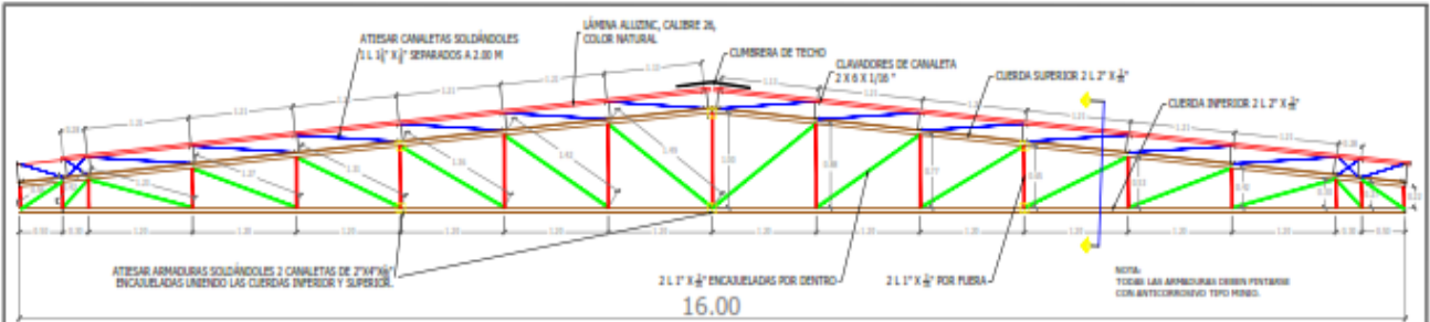
DETALLE DE ARMADURA TIPO A-01
