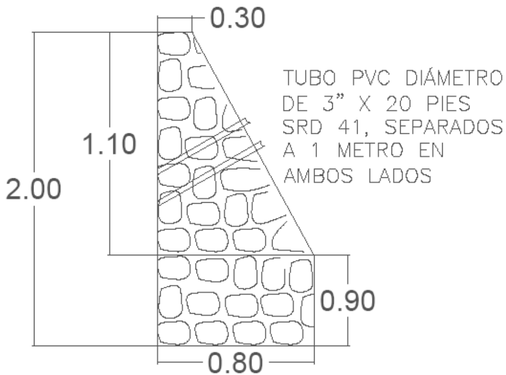
DETALLE DE MURO DE MAMPOSTERIA
