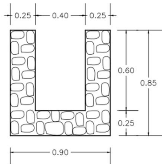
DETALLE CUNETAS MAMPOSTERIA
