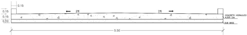
CALLE DE CONCRETO HIDRAULICO sin escuela
