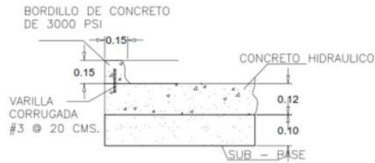
DETALLE BORDILLO DE 15 CM X 15 CM
