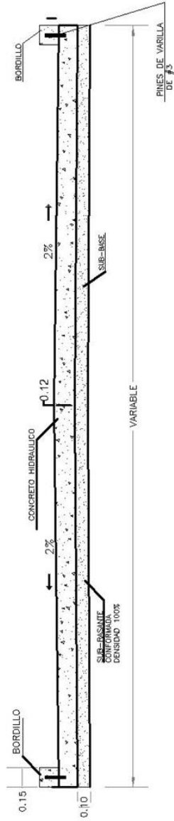
SECCION TIPICA DE CONCRETO HIDRAULICO
