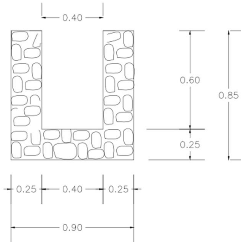
DETALLE CUNETAS DE MAMPOSTERÍA
