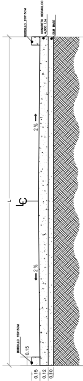
SECCION TIPICA CALLE DE CONCRETO HIDRAULICO
