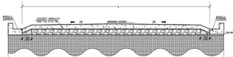
SECCION TIPICA DE WHITE TOPPING
