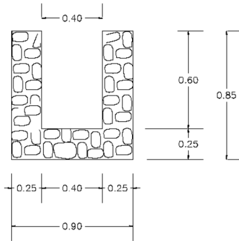
DETALLE CUNETAS DE MAMPOSTERÍA
