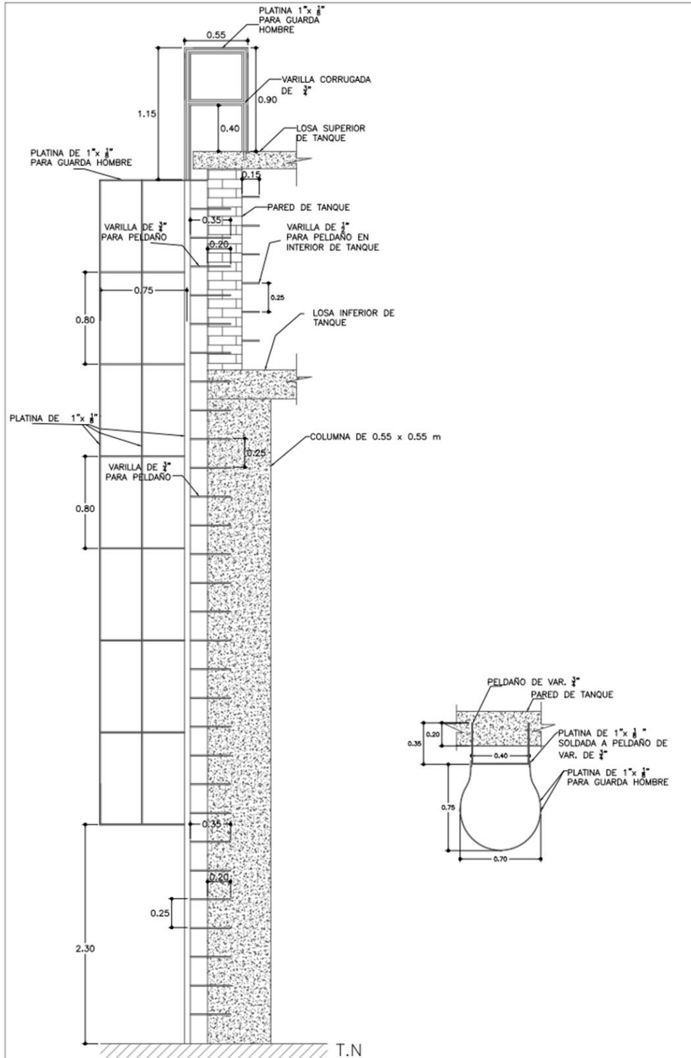
DETALLE DE GRADAS CON GUARDA HOMBRE TANQUE ELEVADO DE 30,000 GALONES
