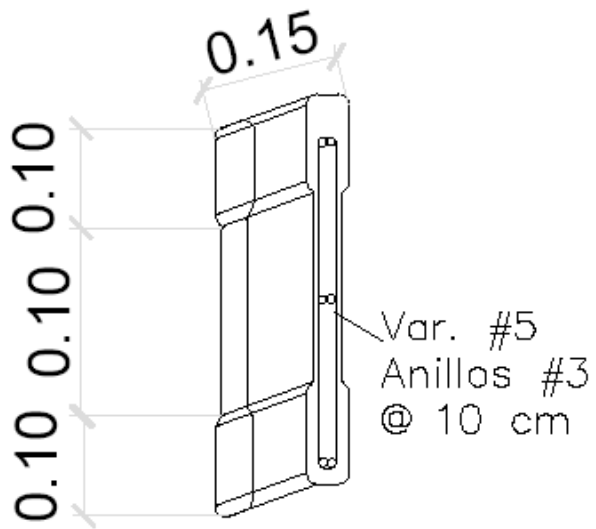
Vista isométrica
