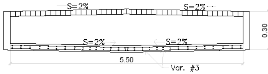
CORTE A-A
