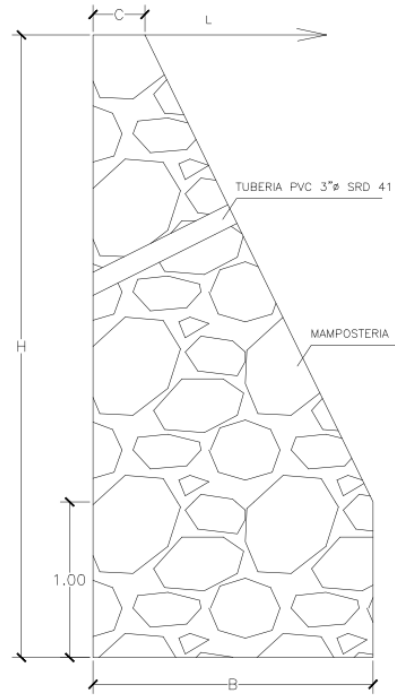
DETALLE DE MUROS DE CONTENCION ESC. 1:100
