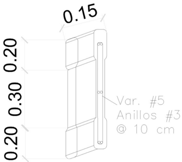
Vista isométrica
