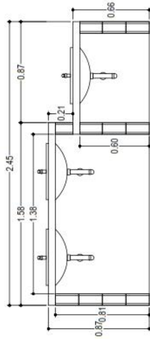
ELEVACIÓN DE LOSA DE LAVAMANOS
