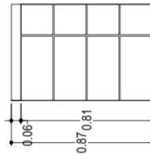
ELEVACIÓN DE MUEBLE DE LAVAMANOS
