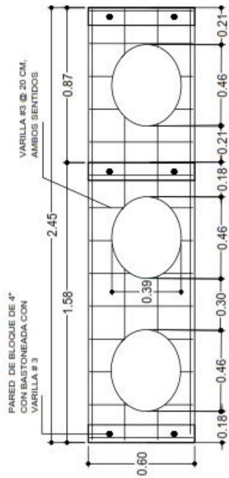
ESTRUCTURA DE LOSA DE LAVAMANOS
