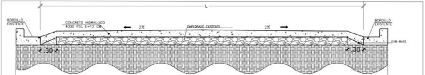
SECCION TIPICA DE WHITE TOPPING
