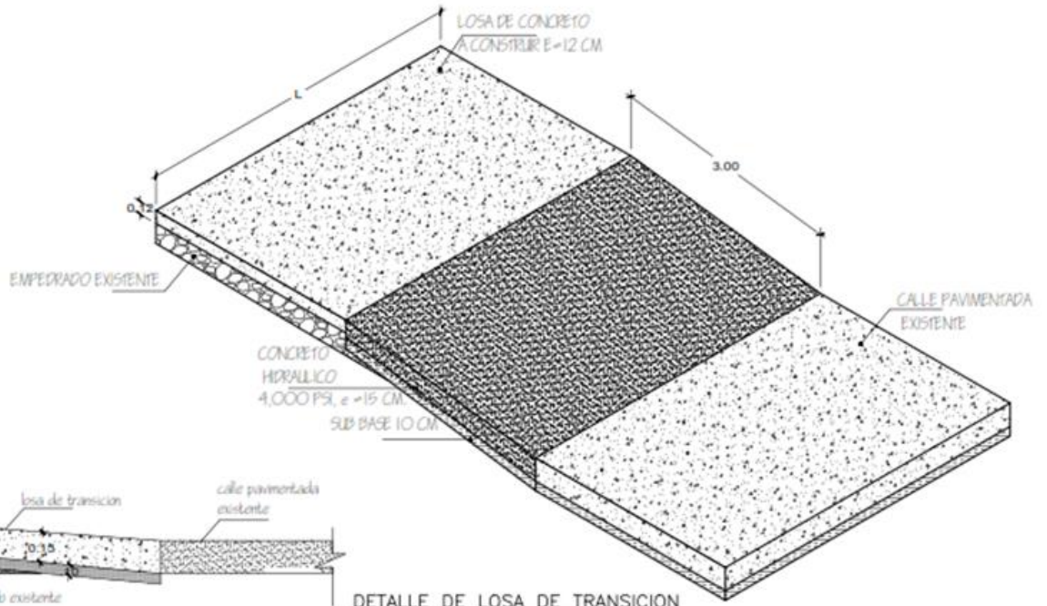
DETALLE DE LOSA DE TRANSICION
