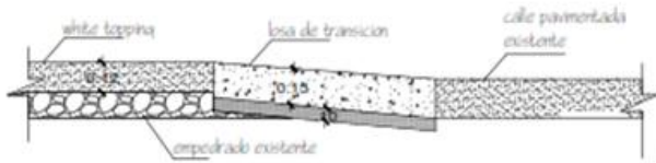
DETALLE DE LOSA DE TRANSICION
