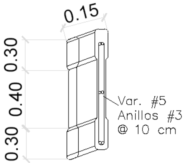
Vista isométrica
