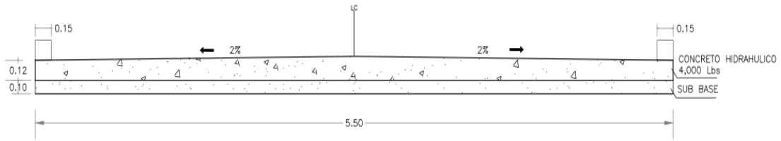
CALLE DE CONCRETO HIDRAULICO sin escala
